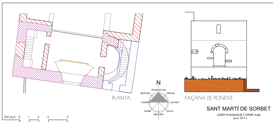
SANT MARTÍ DE SORBET. Planta de l'església integrada com a vestibol de l'actual i façana de ponent.
