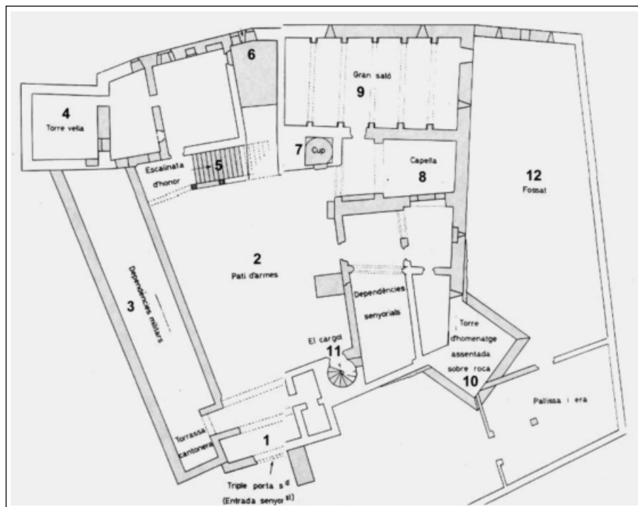
CASTELL DE BELLCAIRE D'EMPORDÀ. Planta extreta de Viquipèdia.
