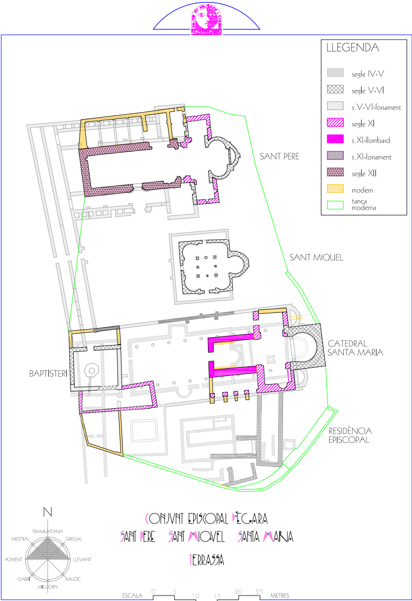
CONJUNT EPISCOPAL D'ÒRGARA. Planta general de les estructures episcopals. Publicada al llibre: La seu episcopal d'Òrgara. Arqueologia d'un conjunt cristià del segle IV al IX , de M. Gemma Garcia Llinares, Antoni Moro Garcia i Francesc Tuset Bertran. Institut Català d'Arqueologia Clàssica. Tarragona, 2009.
