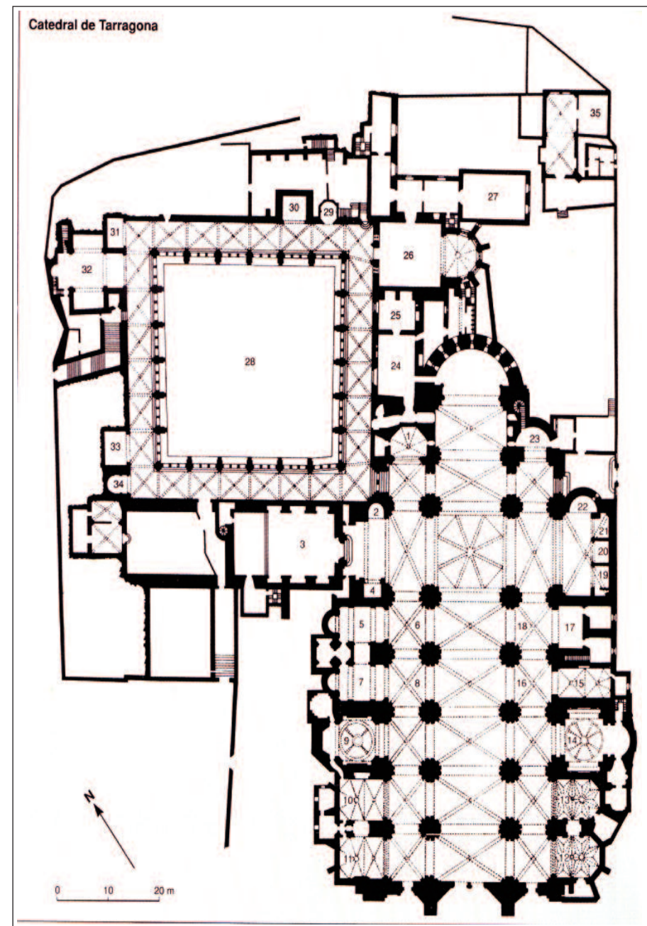
CATEDRAL DE SANTA MARIA. TARRAGONA. Planta de Catalunya Romànica vol. XXI, p.125.
