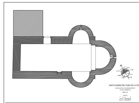
SANTA MARIA DEL PUIG DE LA CREU. Planta.
