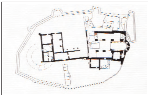
SANT PERE D'ÀGER. Planta del Servei d'arquitectura de la Diputació de Lleida.
