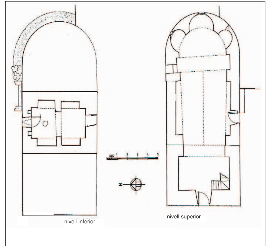
MONESTIR DE SANT POL DE MAR. Planta de J.A. Adell, publicada a Catalunya Romànica, vol. XX, p. 517
