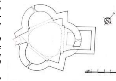
LA MERCÈ DE PLANÈS. Església de planta triangular. Croquis d'A. Adell, extret de la Catalunya Romànica.
