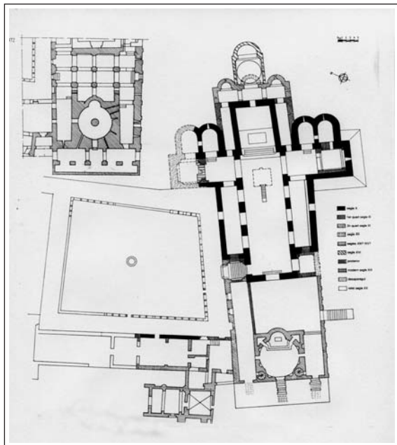
SANT MIQUEL DE CUIXÀ. Els diferents traços equivalen a les diverses etapes de construcció. (Catalunya Romànica, vol. VII).
