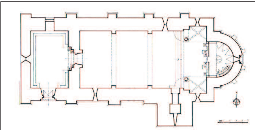
SANTA MARIA DE COSTOJA. Planta de R. Mallol, publicada a Catalunya romànica vol. X, Vallespir, pg. 124.
