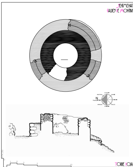
TORRE ROJA. Planta i secció.
