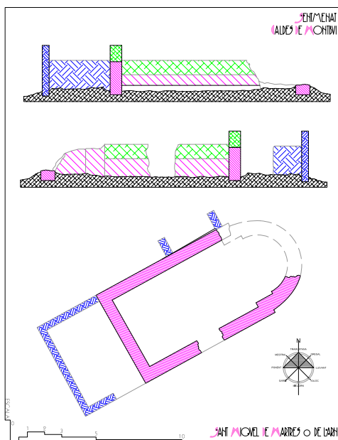
SANT MIQUEL de l'ARN. Planta i seccions.
