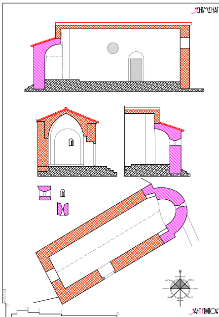
SANT FRUIT S. Planta i seccions.
